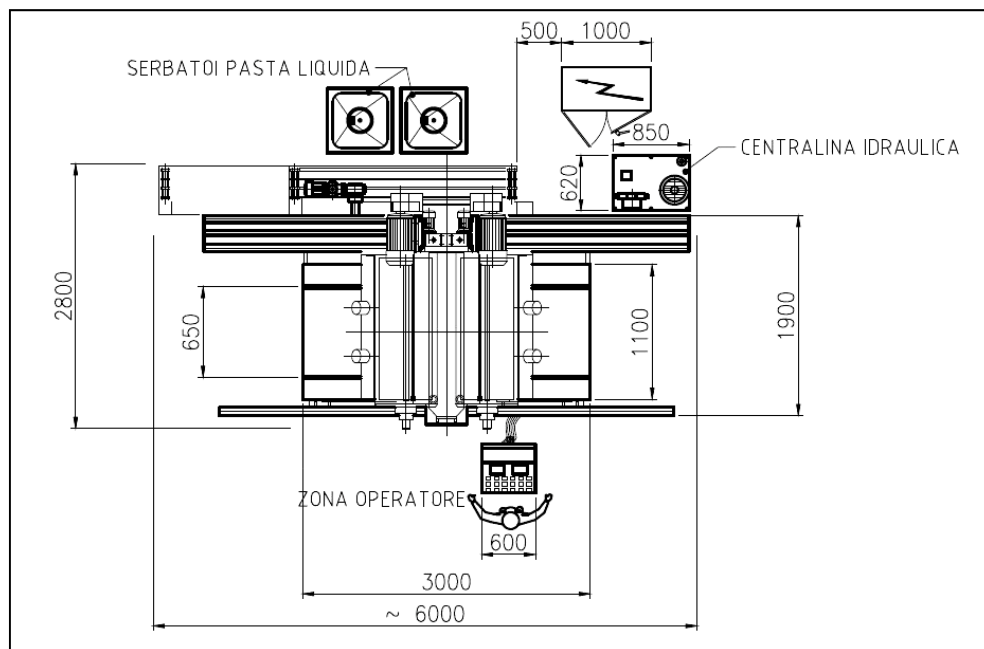
Vista in pianta con ingombri di una macchina Mod. M 600/1100/2UO-3000
